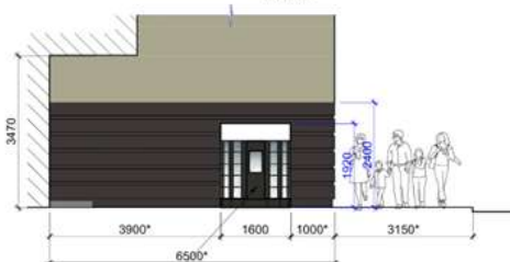
FASĀDES SKATS M1:50
